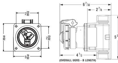
UGRS RECEPTACLE MTG DIMENSIONS
