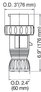
PLUG 20A
